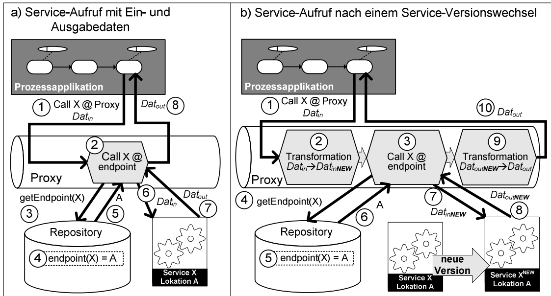
Abbildung 14 Service-Aufruf bei Versionswechsel
