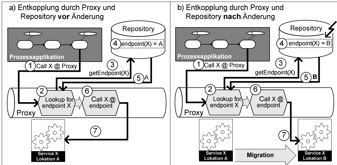
Abbildung 12 Szenarien zur Service-Migration
