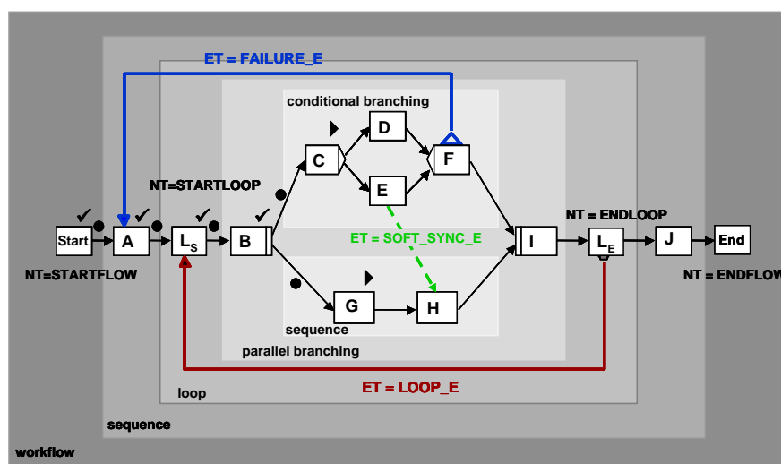
Abb. 7: ADEPT Prozess-Meta-Modell
